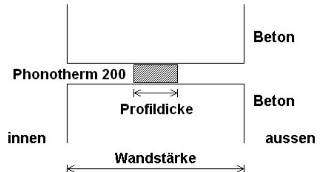
Abb. 2. Phonotherm® 200 – Einbausituation für Wärmeübergang von innen nach außen.
